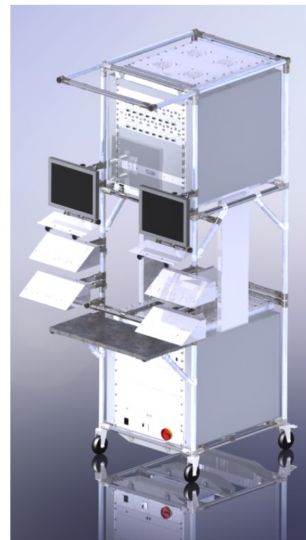
Monipuolinen testilaiteräkki mahdollistaa useiden matkapuhelinten samanaikaisen elektronisen testauksen.
